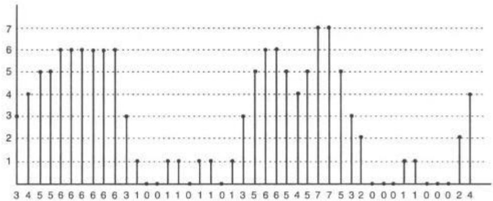
Figuur 1.18 Staafdiagram voor de gedigitaliseerde waarden.
