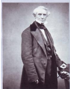
Figuur 1.3 Morse en zijn alfabet.
