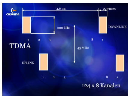
Figuur 2.11 Een TDMA kanaal: elk 8 e tijdslot. Het uplink-tijdslot 1 loopt een paar tijdsloten achter op het downlink-tijdslot 1.
